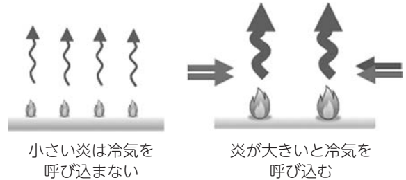
図1 炎の大きさによる違い
