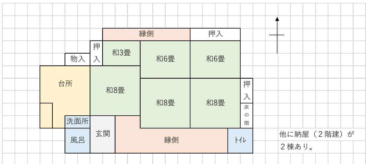
間取り図 (イメージ)
